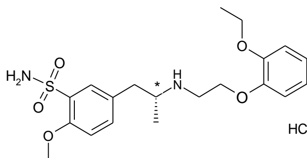
Tamsulosin hydrochloride:
