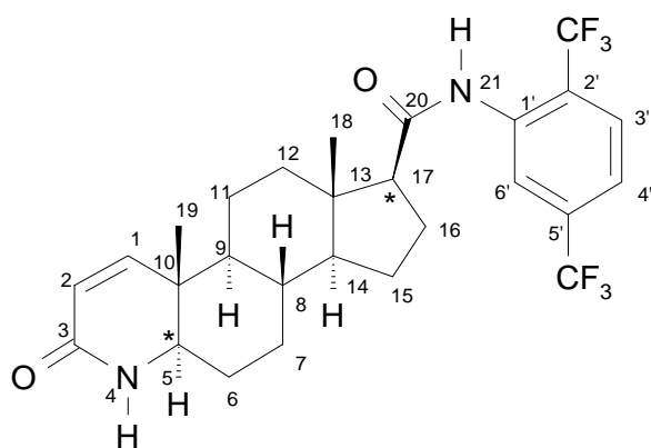
Dutasteride:
